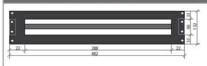
Dimensiones perfil omega
