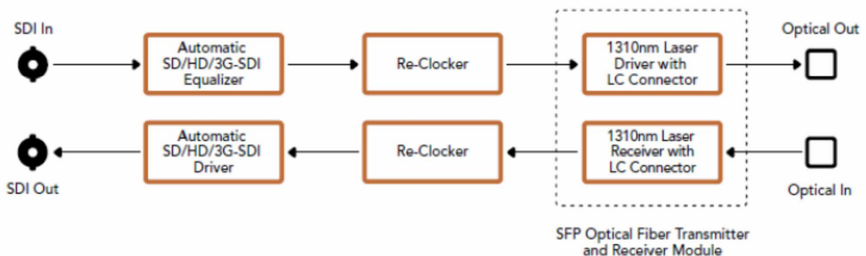
Mini Converter Optical Fibre Block Diagram
