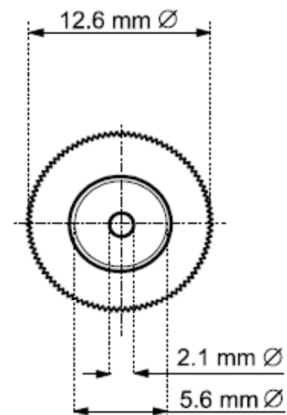
Vorderansicht front view
