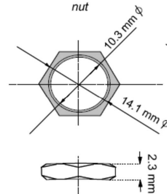
Mutter nut
