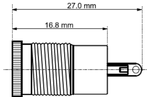
Seitenansicht side view
