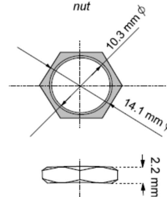
Mutter nut
